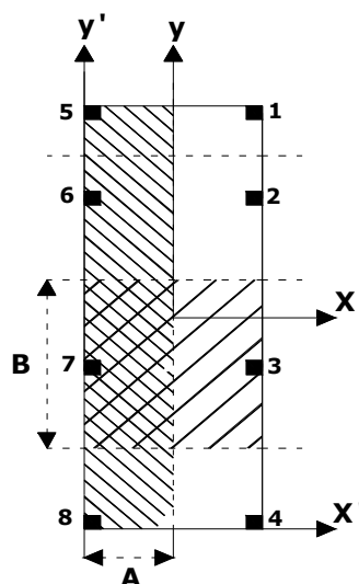
شکل ۱-۷- نوارهای بحرانی پی
