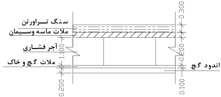
شکل ۱-۱۴ - جزئیات پاگرد
