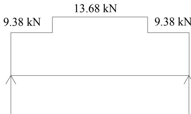
شکل ۵-۱- نمایش نیروی برشی وارد بر پله
