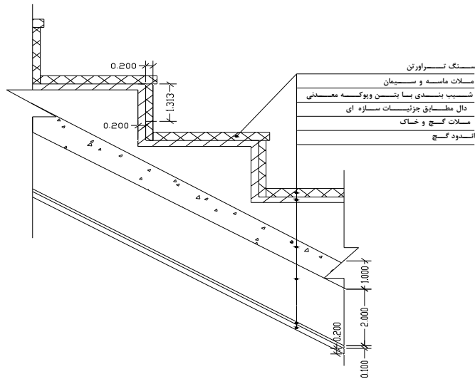
شکل ۱-۱۳ - جزئیات پله
