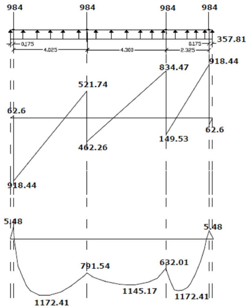
شکل ۷-۲- نمایش نیروهای وارده و نمودار لنگر خمشی و نیروی برشی
