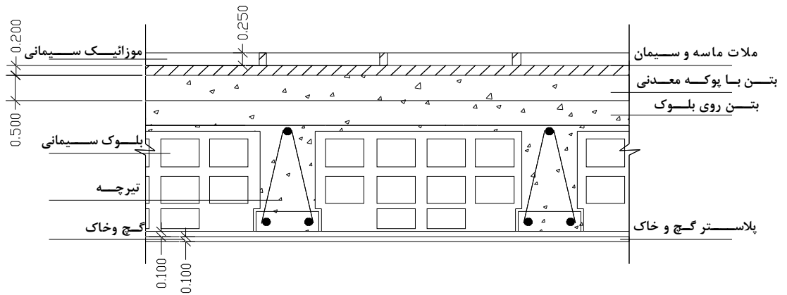
شکل ۱-۱-۱۱ - جزئیات سقف طبقات
