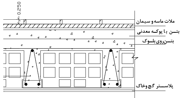
شکل ۱-۱- جزئیات سقف بام
