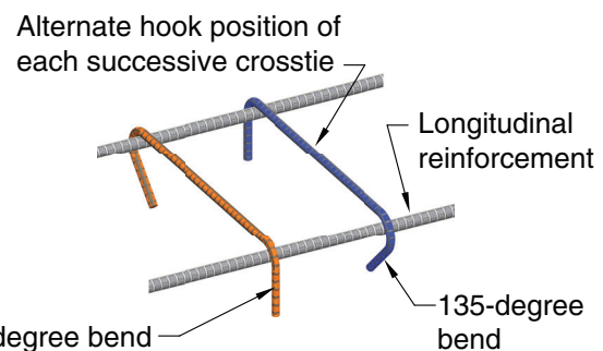
Fig. R25.3.5—Crosstie.
