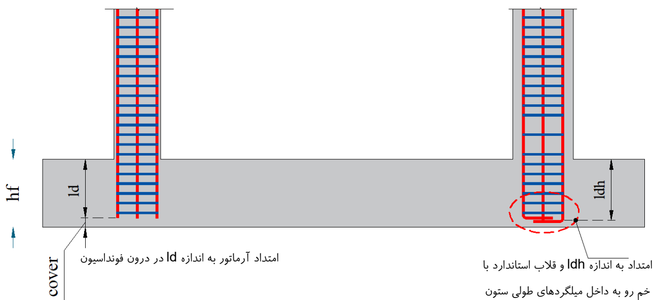
شکل ۳-۸: محدودیت امتداد میلگردهای طولی ستون در فونداسیون
