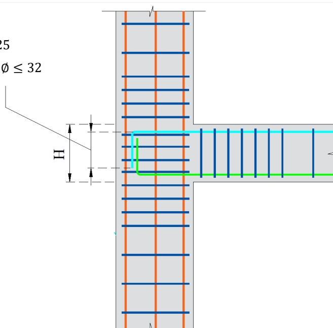
شکل ۵-۲: محدودیت ارتفاع تیر برای امکان تعبیه قلاب میلگرد طولی
