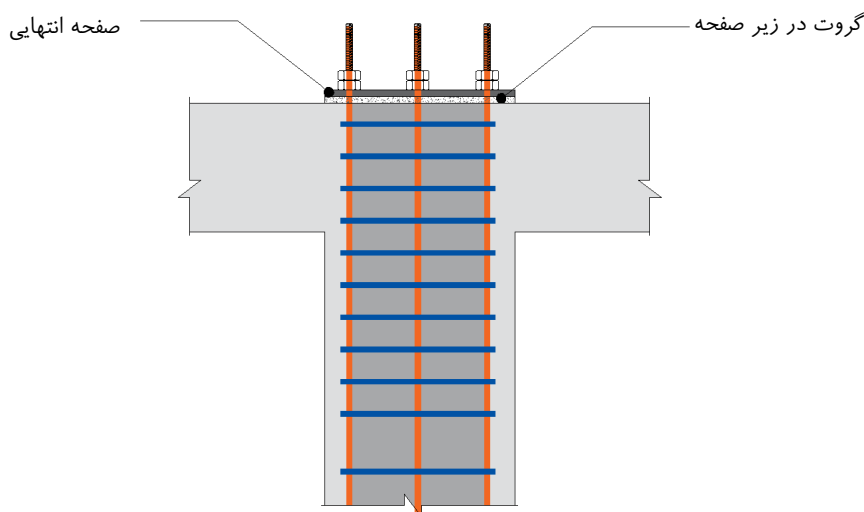
شکل ۳-۱۶: مهار میلگردهای طولی با استفاده از صفحه انتهایی
