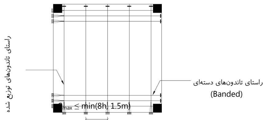
شکل ۷-۵: حداکثر فاصله تاندون‌ها در راستای توزیع شده (Distributed)
