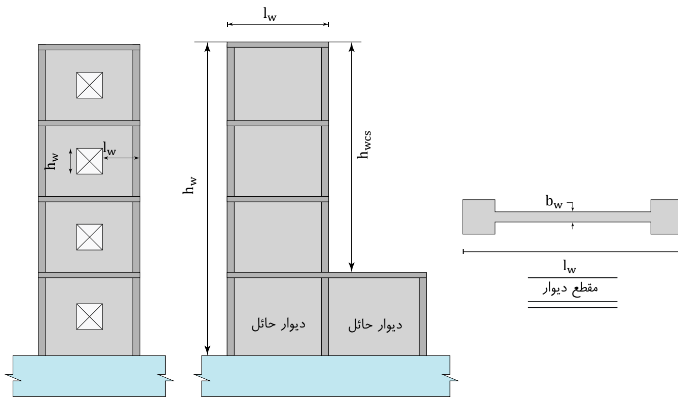
شکل ۴-۵۱: نمایش پارامترهای l_w و h_w مربوط به دیوار بدورن بازشو و دیوار دارای بازشو
