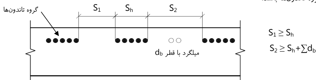
شکل ۵-۲۶: حداکثر فاصله تاندون‌ها در راستای توزیع شده (Distributed)
