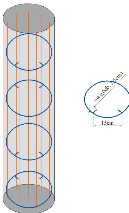
شکل ۱۱-۳: دورگیرها در ستون با مقطع دایره
