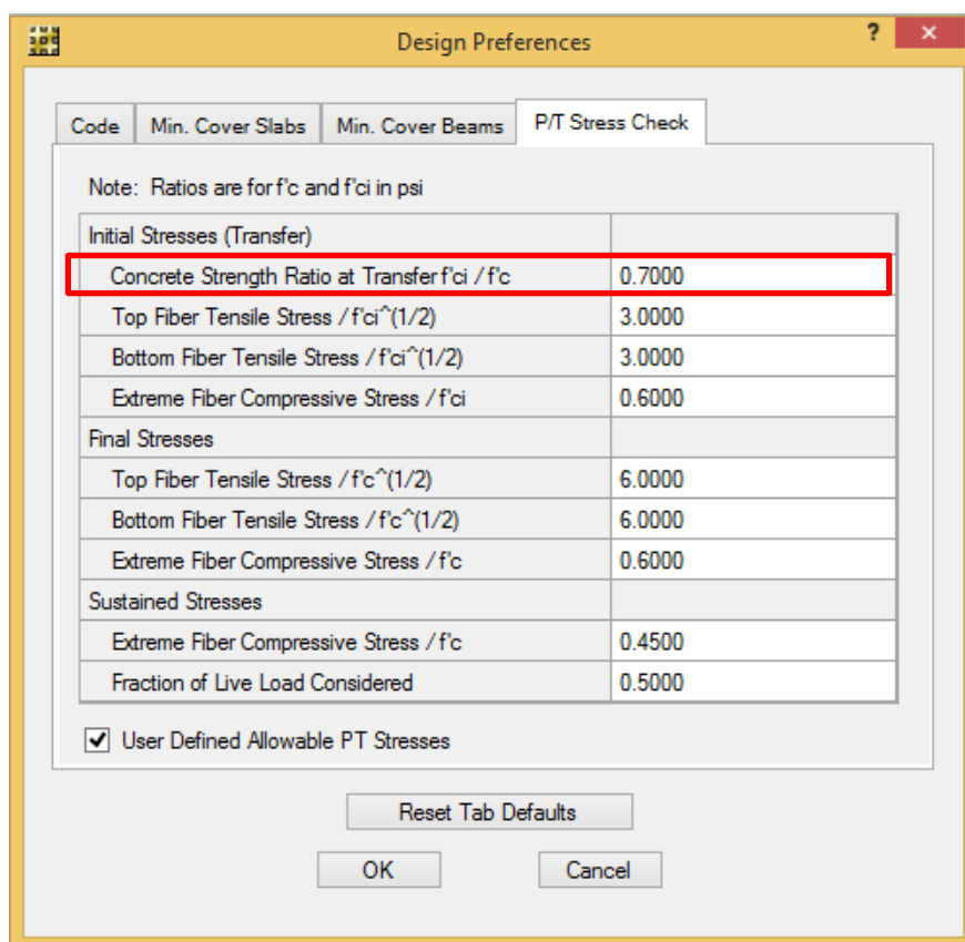
شکل ۵-۳۰: تنظیمات مربوط به نسبت مقاومت اولیه بتن به مقاومت ۲۸ روزه آن در دال‌های پس کشیده
