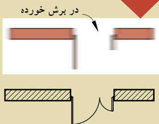
شکل ۳-۹۹ مرحله‌ی سوّم (پلان دیوار و در دولنگه)
