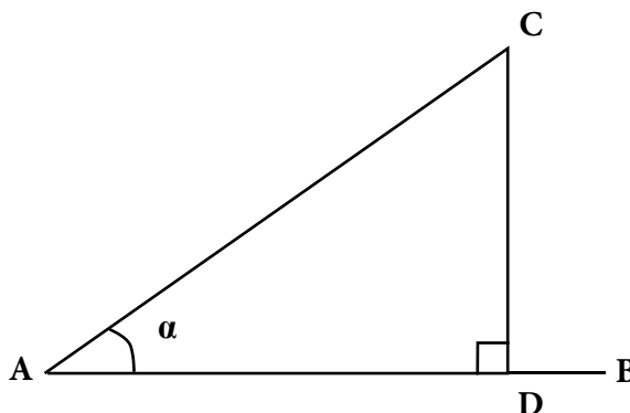
شکل ۴-۱۸. پیاده کردن زاویه نامشخص با متر
