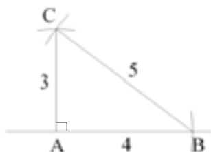
شکل ۴-۱۷. پیاده کردن زاویه عمود با متر (روش ۳-۴-۵)
