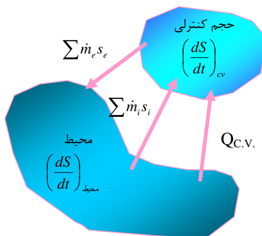
شکل ۵-۳۶. تبادل گرما و آنترופی بین سیستم و محیط
